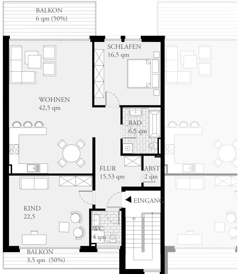
Grundriss (ohne Maßstab)
